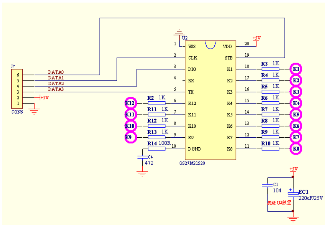
图7-1 GRM807ES_11应用电路
