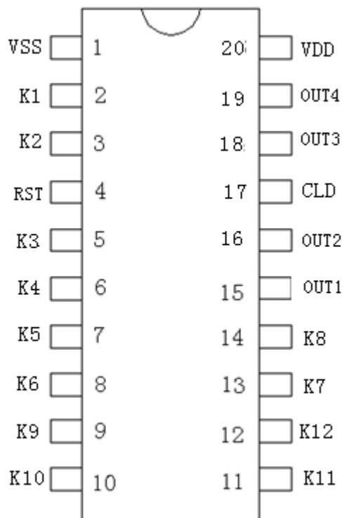
图5-1 GRM810S_11 管脚图
