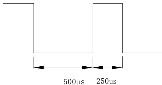
图 8-2 主板向面板发送“1”的定义
