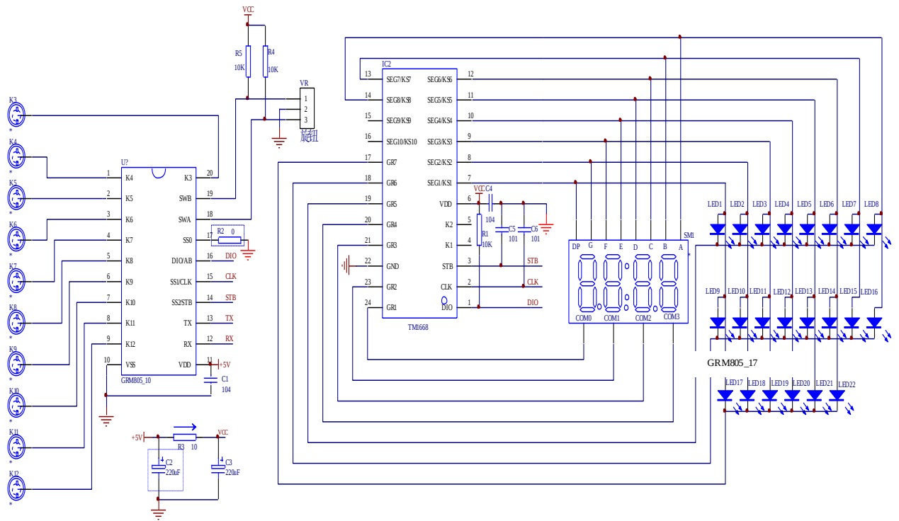
图6-4 GRM805_17触摸键配合16X8显示应用电路
