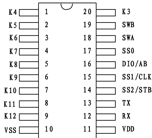
图5-1 GRM805_17 管脚图
