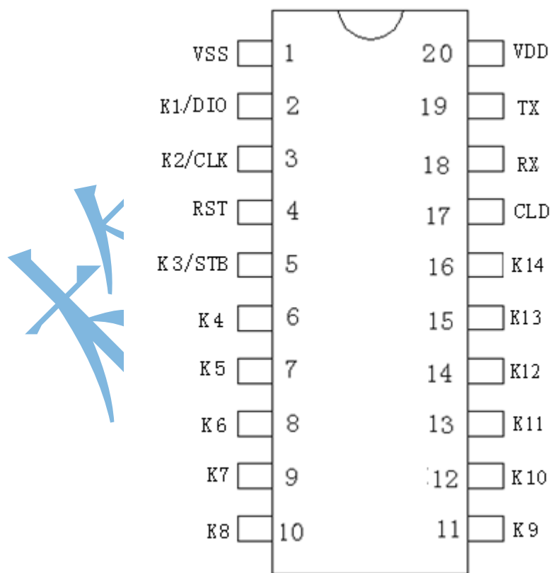
图 5-1 GRM810S_14 管脚图
