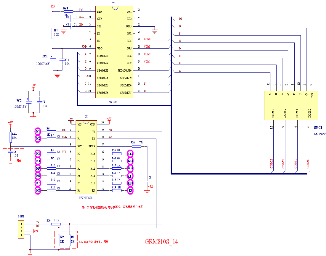
图11-1 GRM810S_14应用电路
