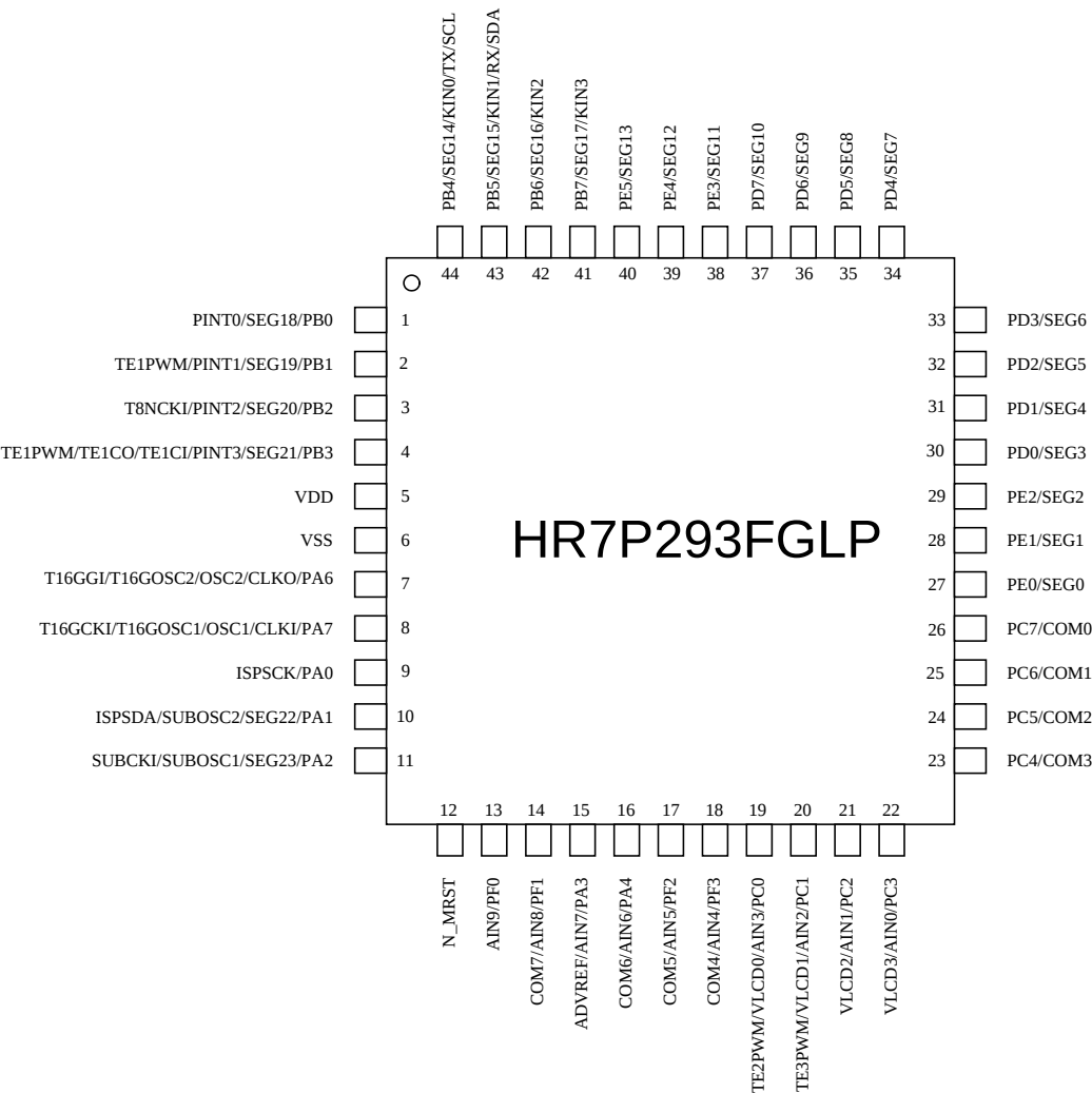
图 1-2 HR7P293FGLP 顶视图
