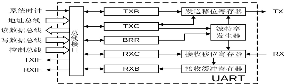
图 5-13 UART 内部结构图
