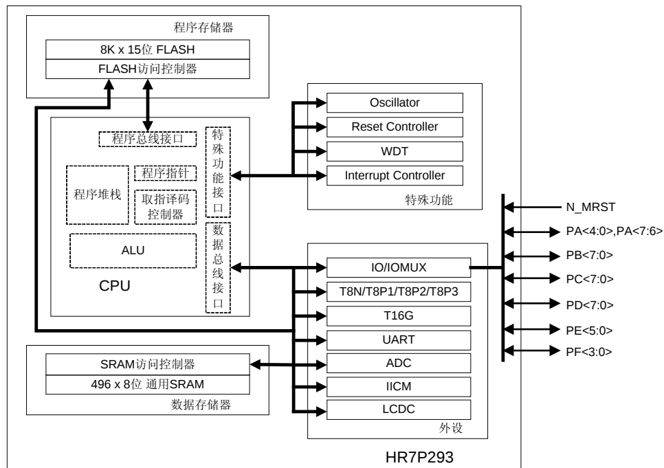
图 1-1 HR7P293 结构框图
