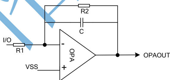
图 6-35 运放应用示意图
