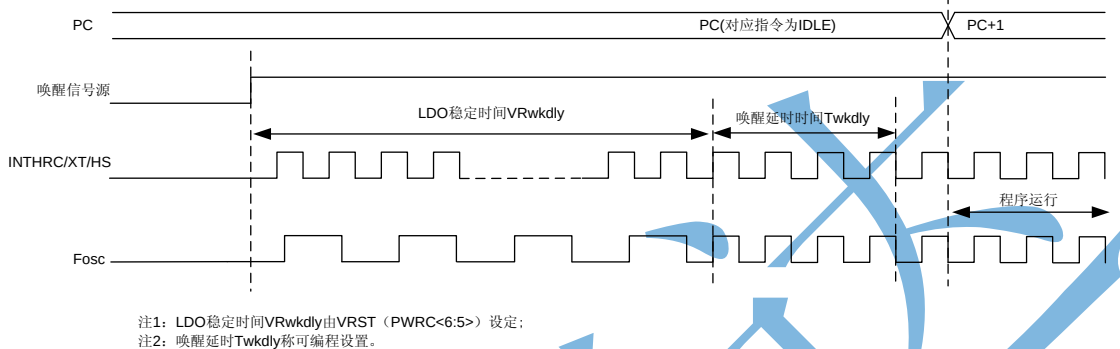
图 5-13 系统时钟为 INTSRC/HS/XT 时，系统唤醒 IDLE0 的时序图
