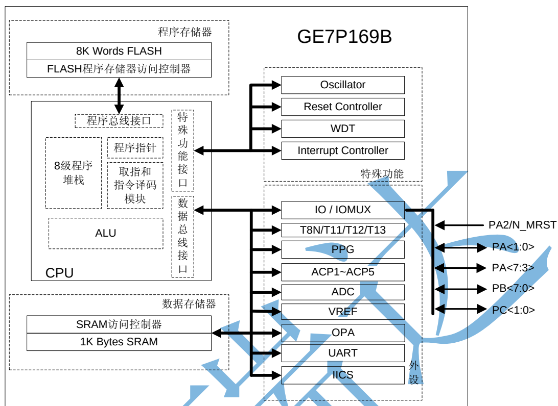
图 1-1 GE7P169B 结构框图
