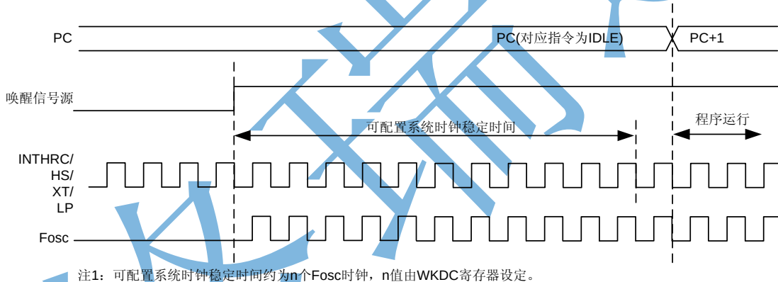
图 5-14 系统时钟为 INTSRC/ LP/HS/XT 时，系统唤醒 IDLE1 的时序图
