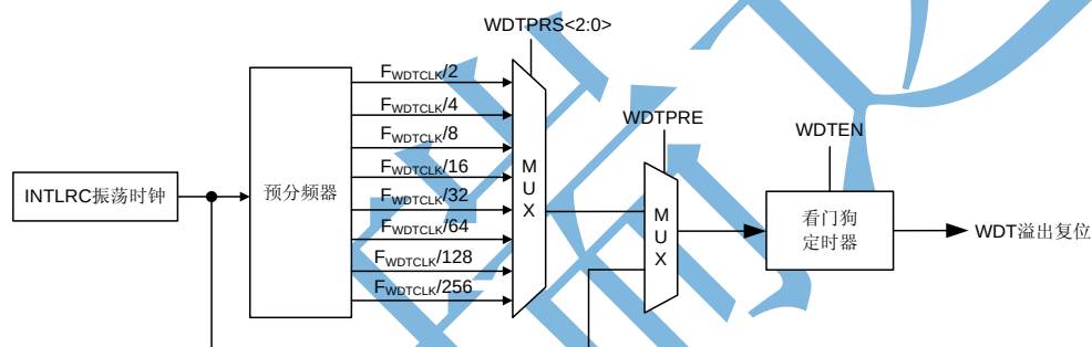
图 5-3 看门狗定时器内部结构图
