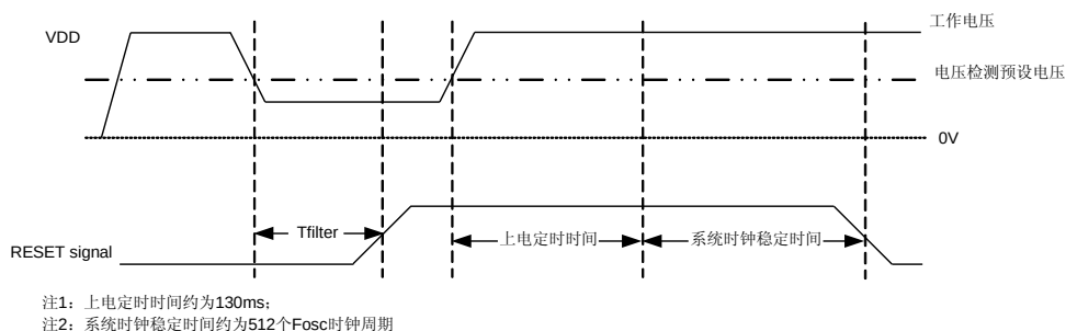
图 5-6 低电压复位时序示意图
