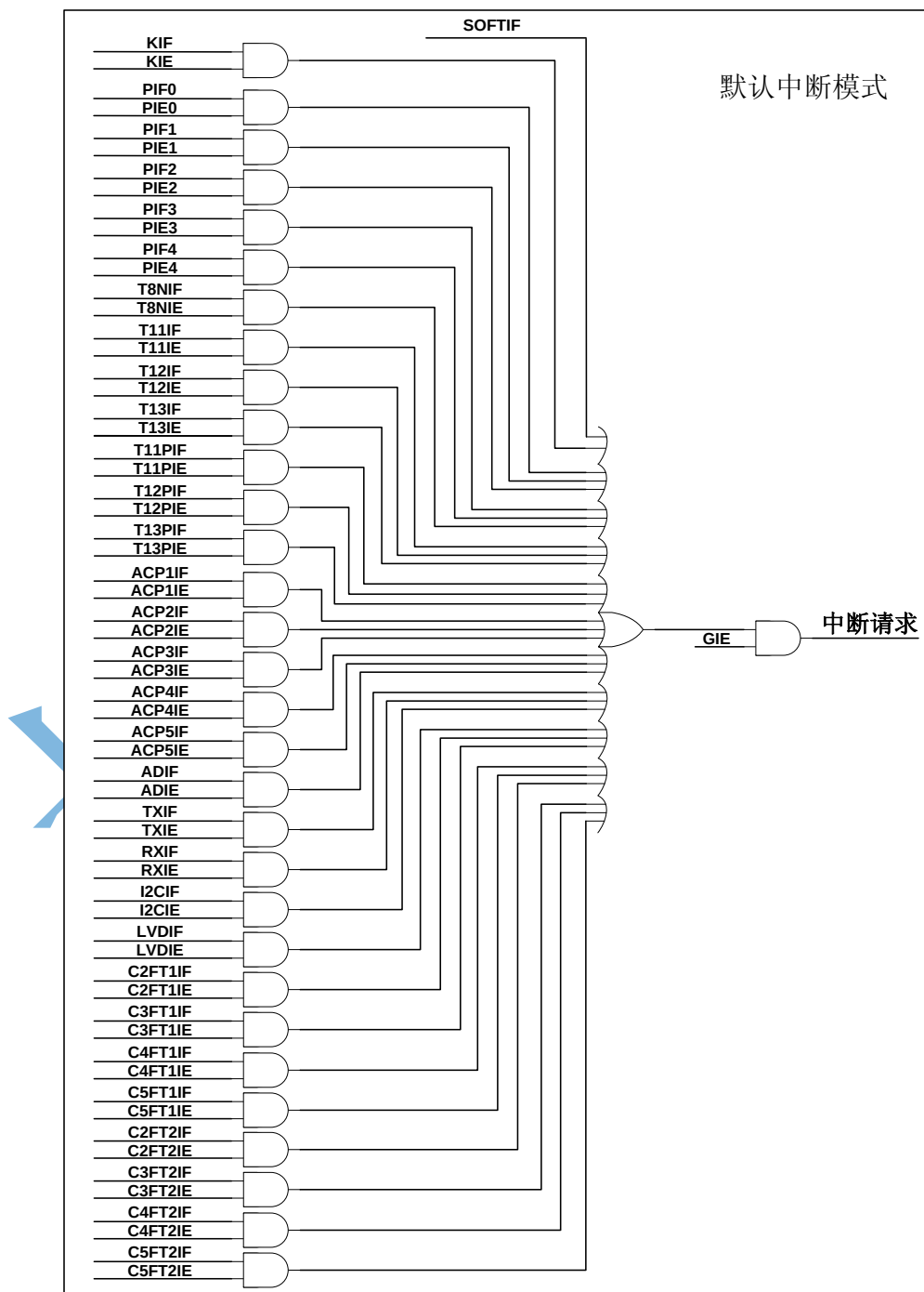
图 7-1 默认中断模式中中断控制逻辑
