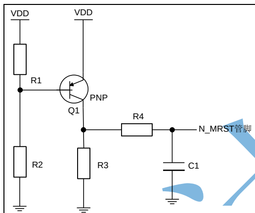
图 5-9 N_MRST 复位参考电路图 2
