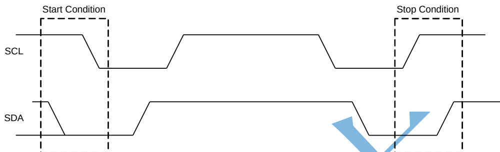
图 6-24 I2C 起始位和停止位
