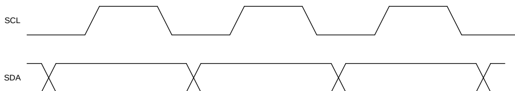
图 6-23 I2C 从动波形图
