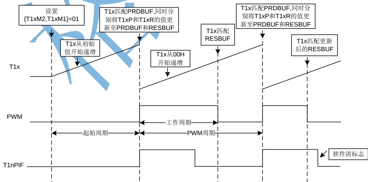
图 6-10 PWM 输出模式示意图
