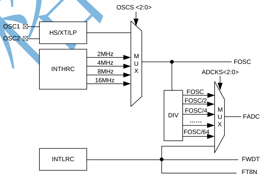
图 5-1 系统时钟结构图
