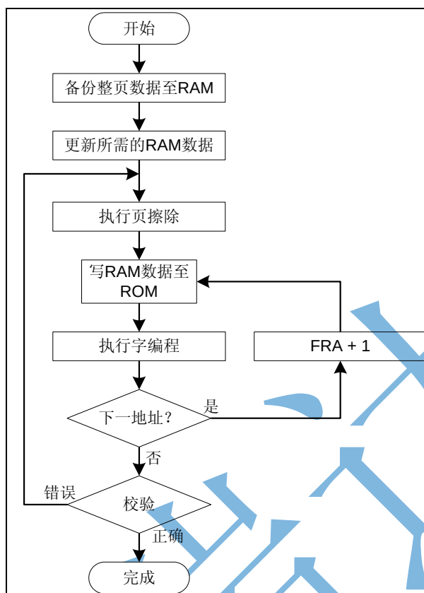
图 3-3 页更新参考流程图
