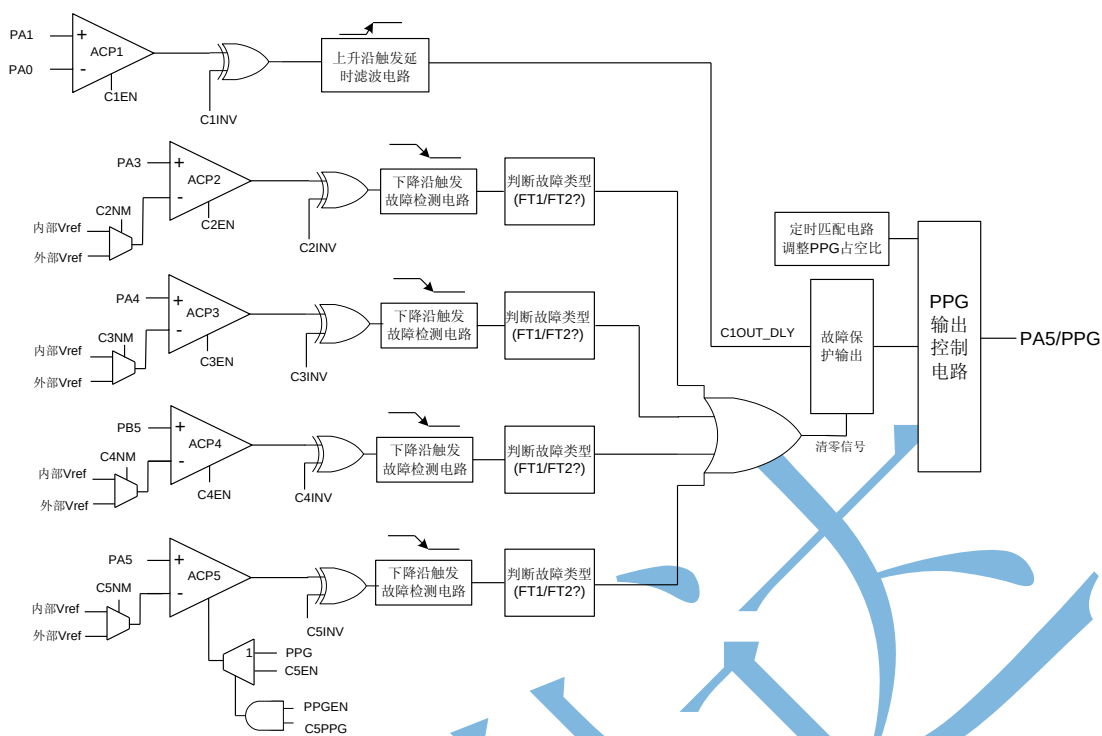
图 6-30 PPG 内部结构图
