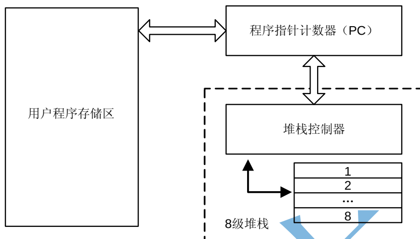
图 3-2 堆栈示意图
