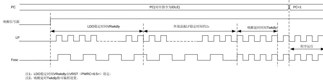
图 5-12 系统时钟为外部 LP 时，芯片唤醒 IDLE0 的时序图
