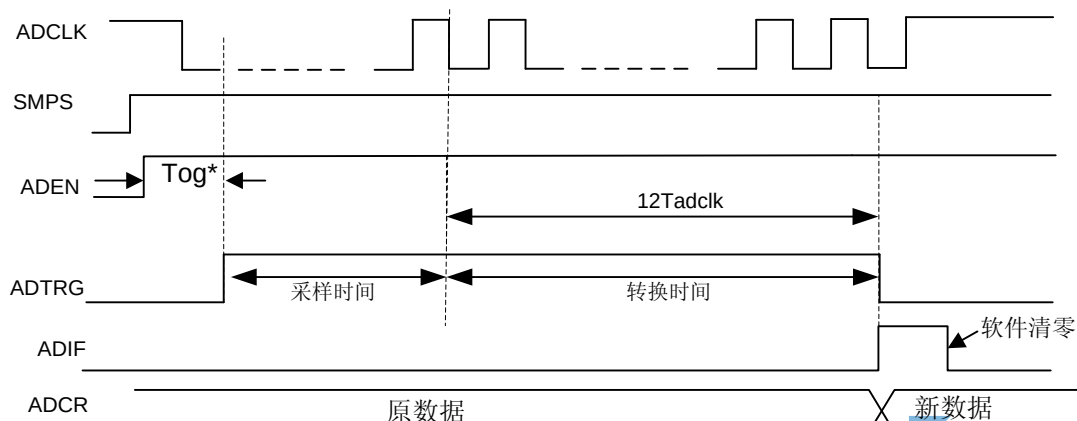
图 6-38 ADC 时序特征示意图 (SMPS=1)
