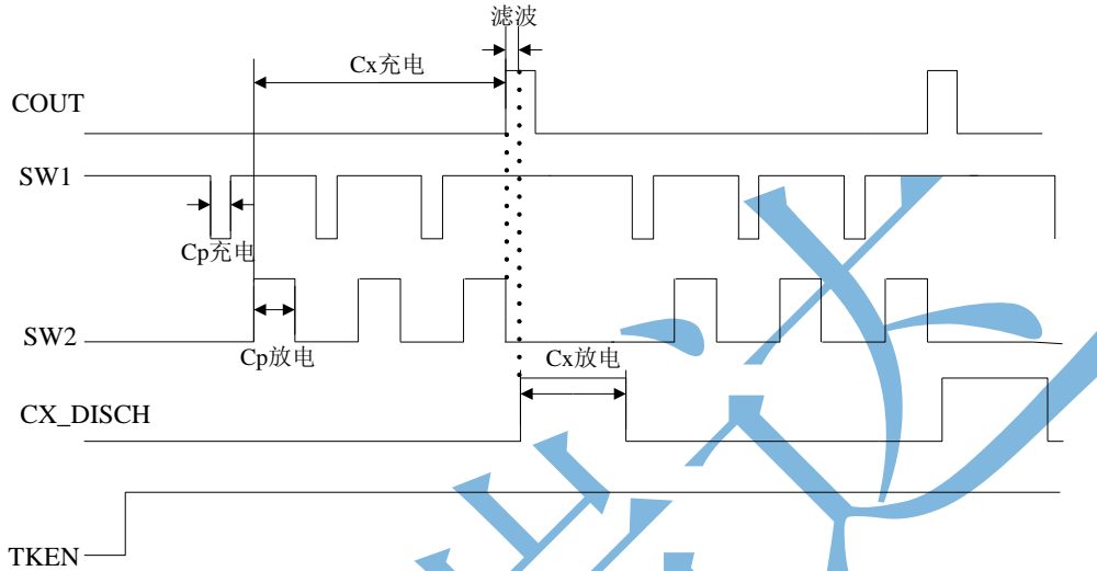
图 5-10 无触摸状态示意图
