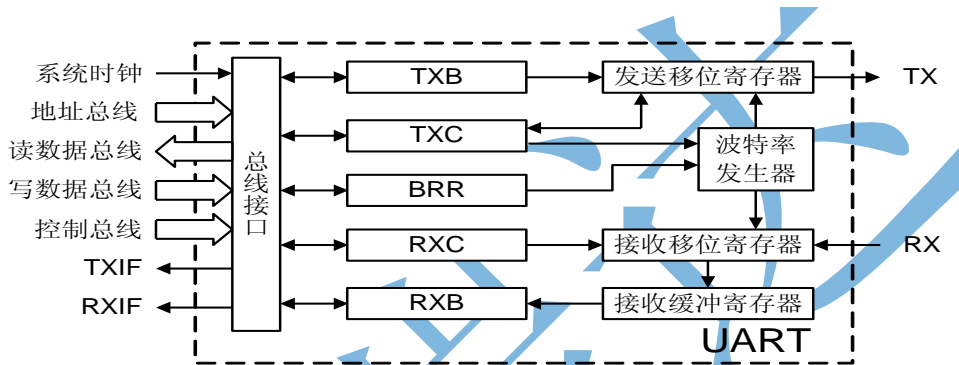
图 5-13 UART 内部结构图
