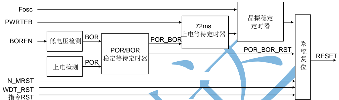
图 6-4 芯片复位原理图
