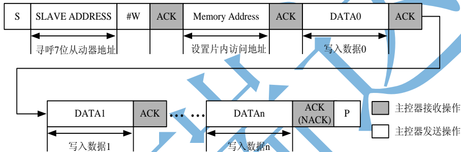
图 5-18 主控器写入从动器数据示意图
