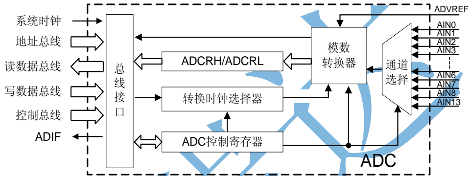
图 5-20 ADC 内部结构图
