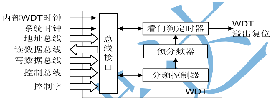
图 6-3 看门狗定时器内部结构图
