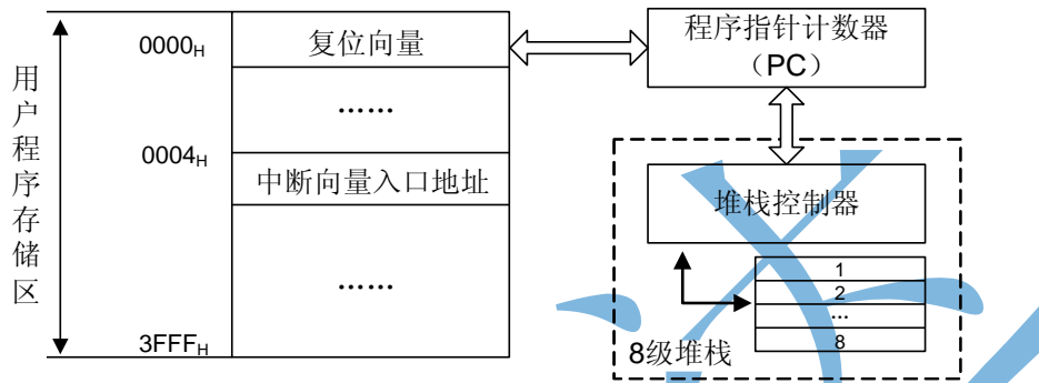
图 3-1 程序区地址映射和堆栈示意图
