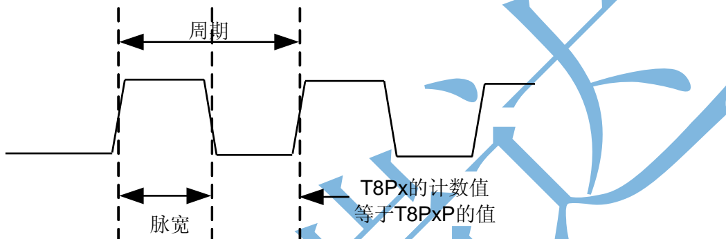
图 5-4 标准 PWM 输出示意图
