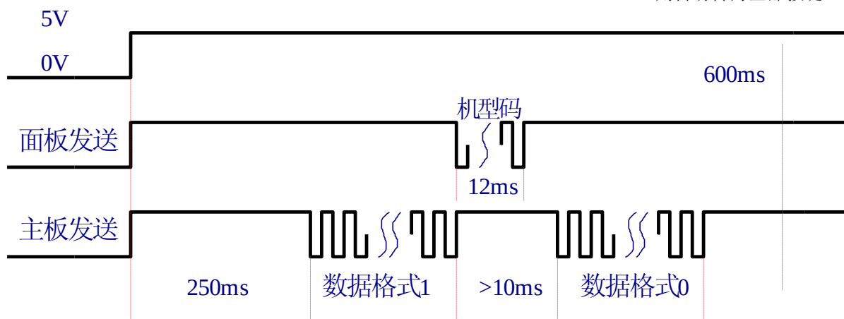
图 10-1 逻辑时序
