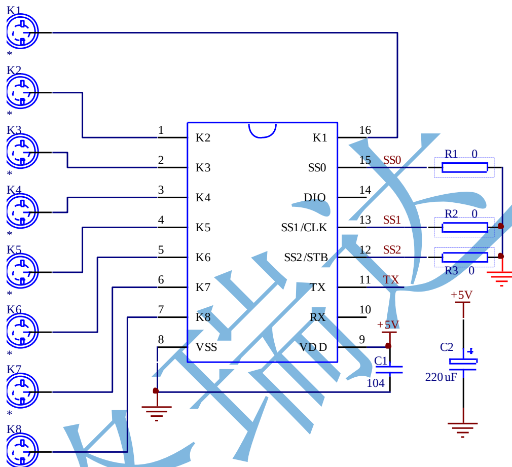
图6-1 GRM805_02作为纯触摸键应用电路
