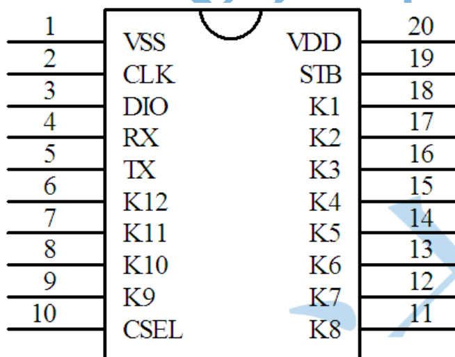
图4-1 GRM807FS_10管脚图
