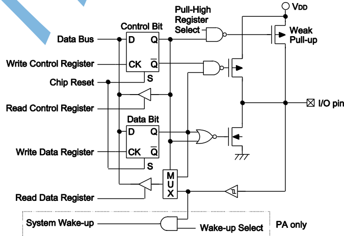
通用输入/输出端口结构
