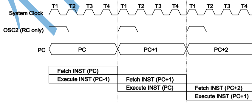
指令捕捉
